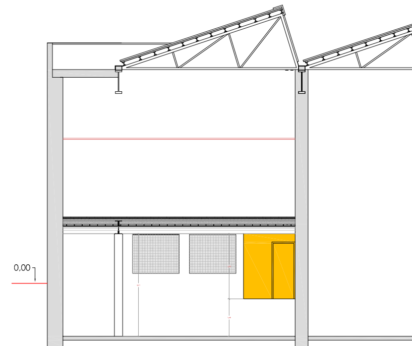
Secció B-B'
