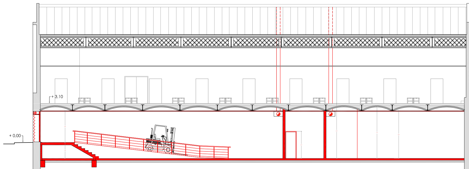
Secció A-A'
