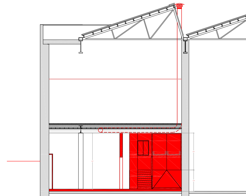
Secció B-B'
