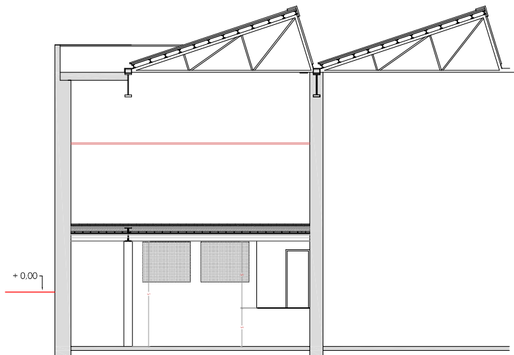
Secció B-B'
