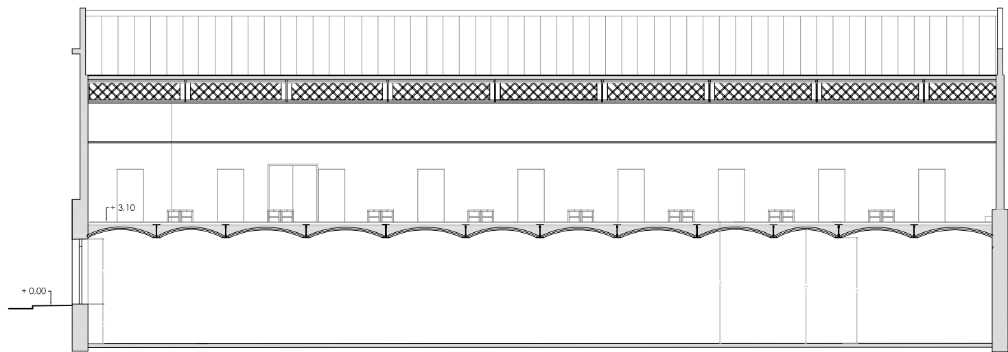
Secció A-A'
