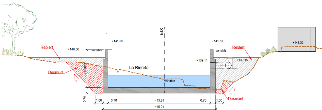
Figura 9. Secció transversal amb moviments de terres per adequació a la proposta
