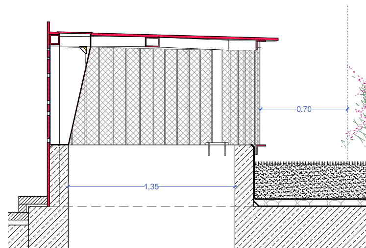
SECCIÓ E 1:30
