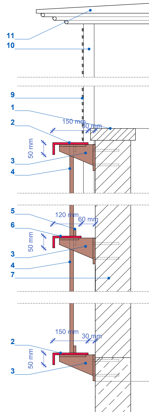
SECCIÓ E 1:10
