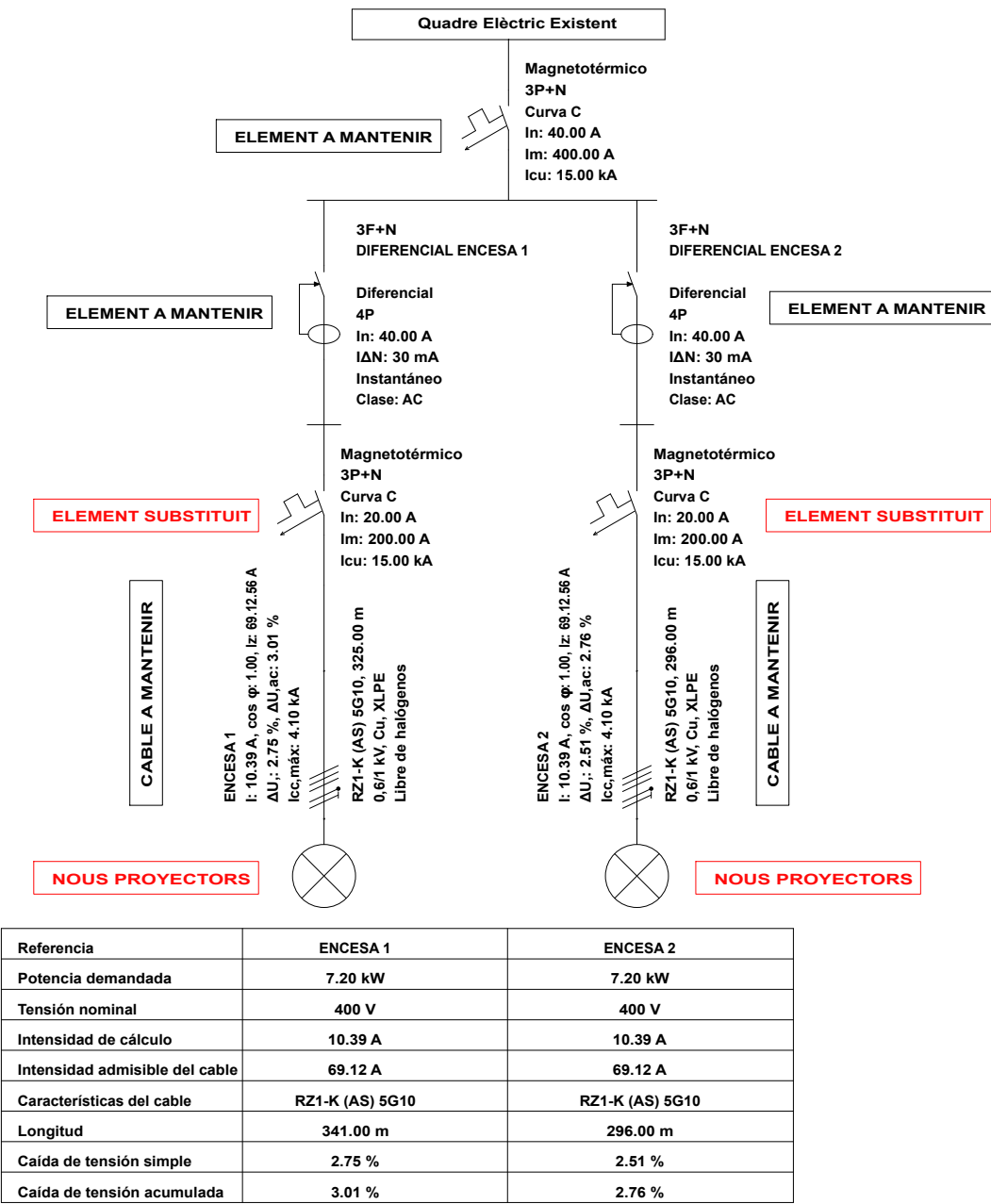
NOVES ENCESES LLUMS CAMP DE FUTBOL
