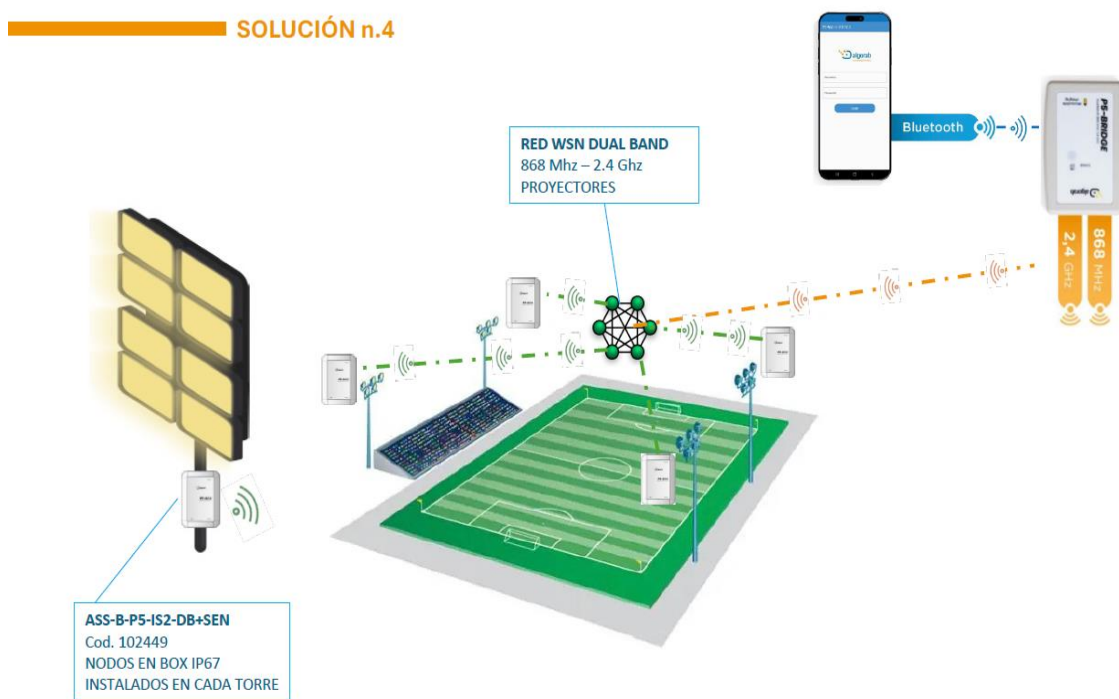
Il·lustració 13. Sistema de control
