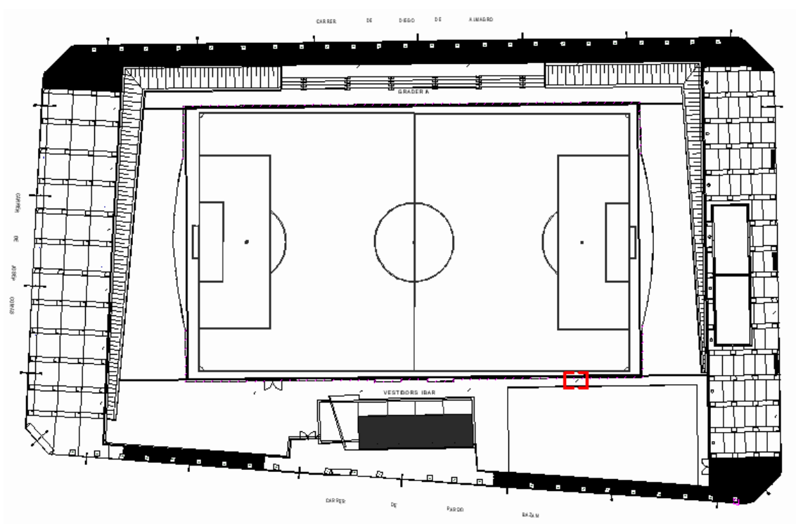
Il·lustració 12. Ubicació columna
