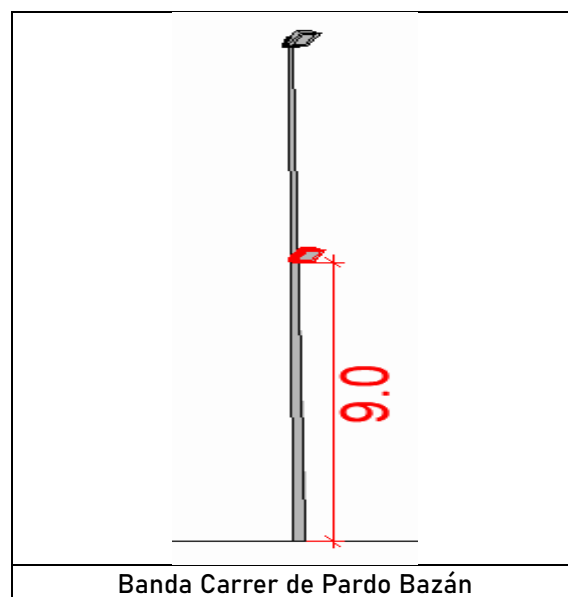
Il·lustració 11. Alçada torre de suport camp d'entrenament
