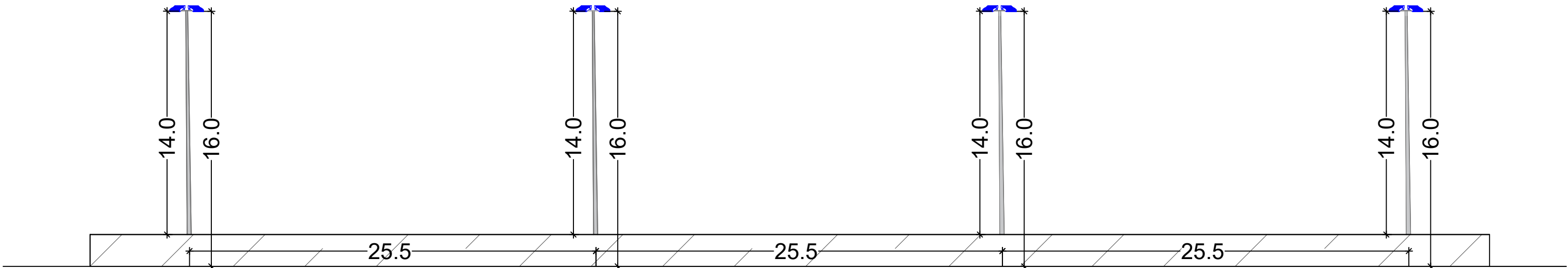
SECCIÓ A-A'
