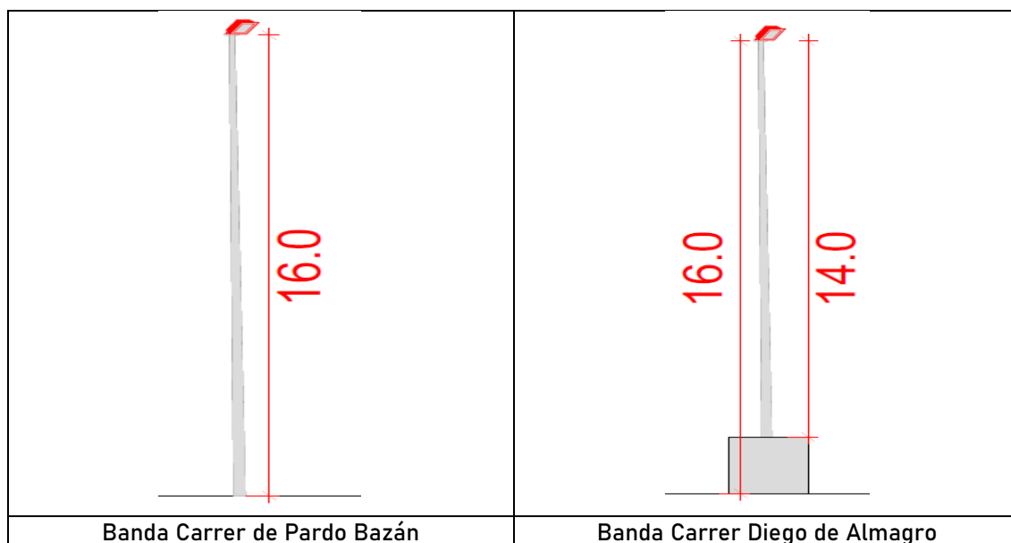
Il·lustració 7. Alçada torres de suport camp futbol
