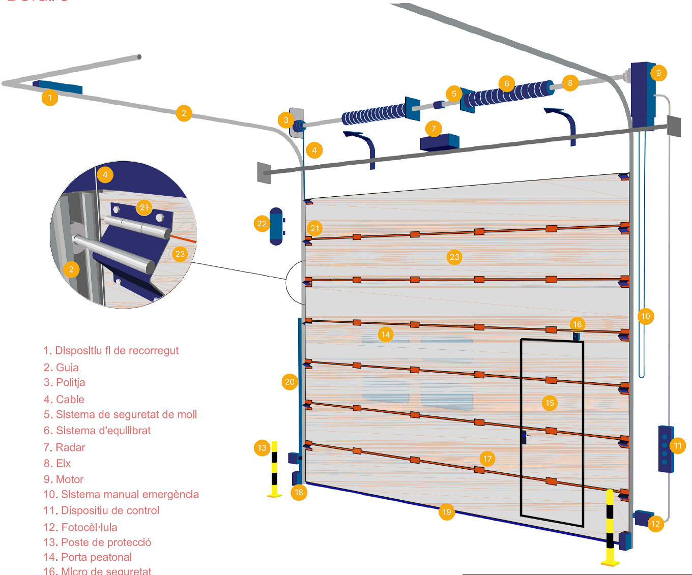
Detall 5
