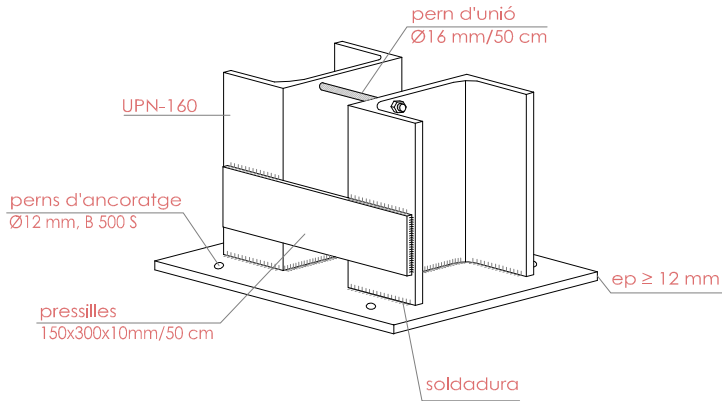
Detall 8
