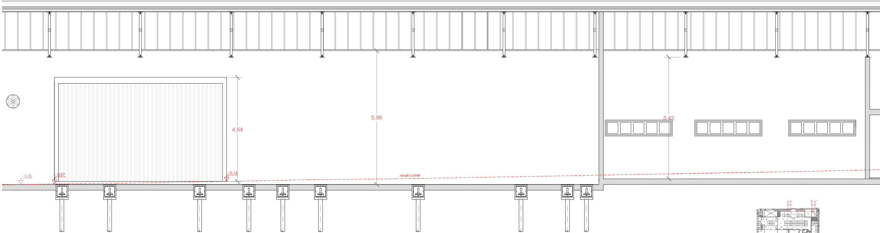
Secció B-B'
