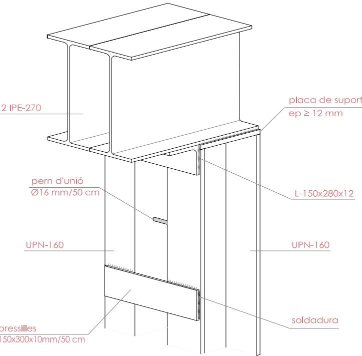
Detall 8
