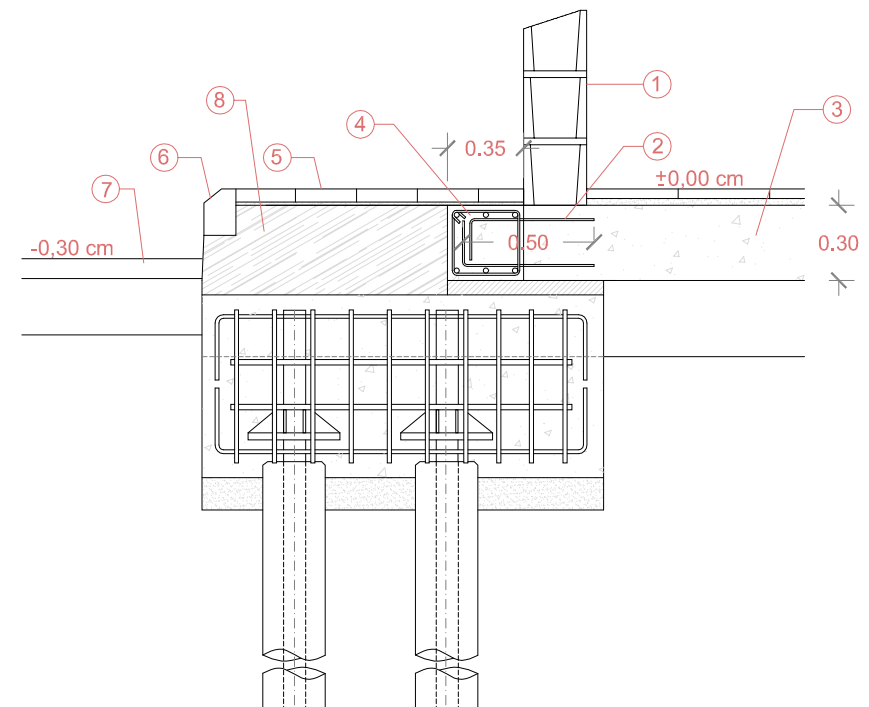
Detall 1
