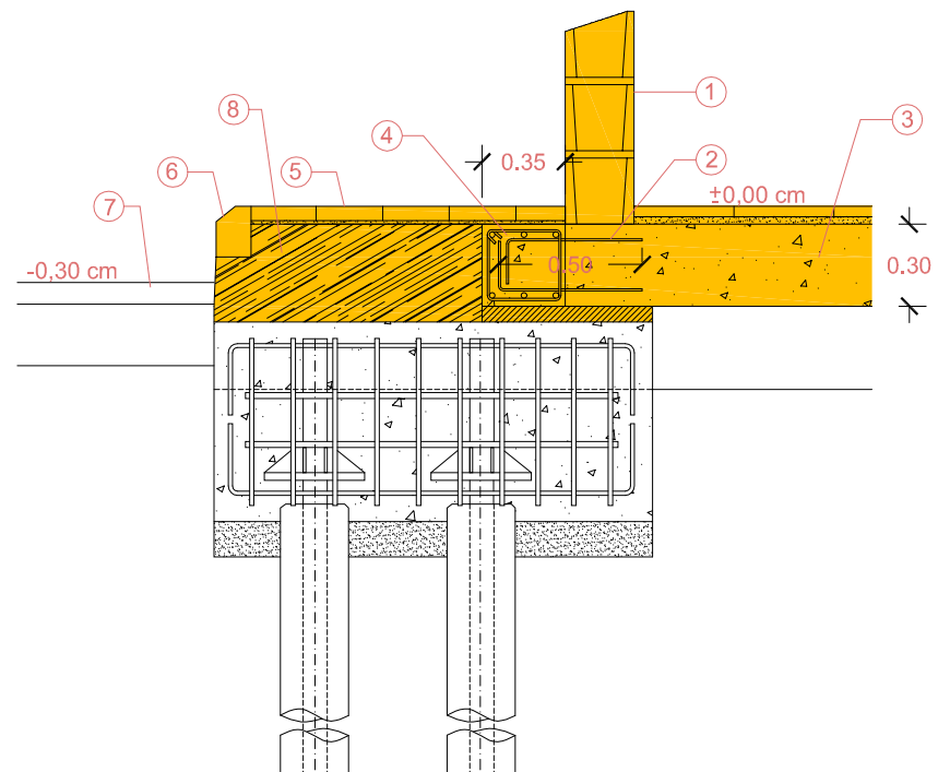
Detall 1
