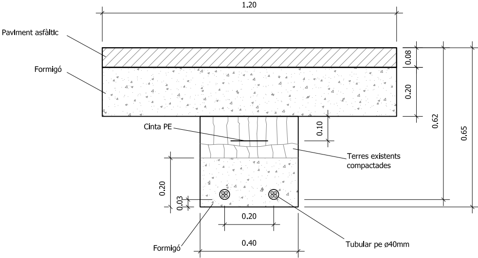
CANALITZACIÓ TIPUS 2 CALÇADA (TUB FORMIGONAT)
