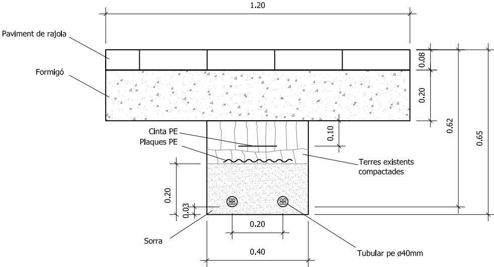
CANALITZACIÓ TIPUS 1 VORERA (PANOT I LLAMBORDA) (TUB SEC)
