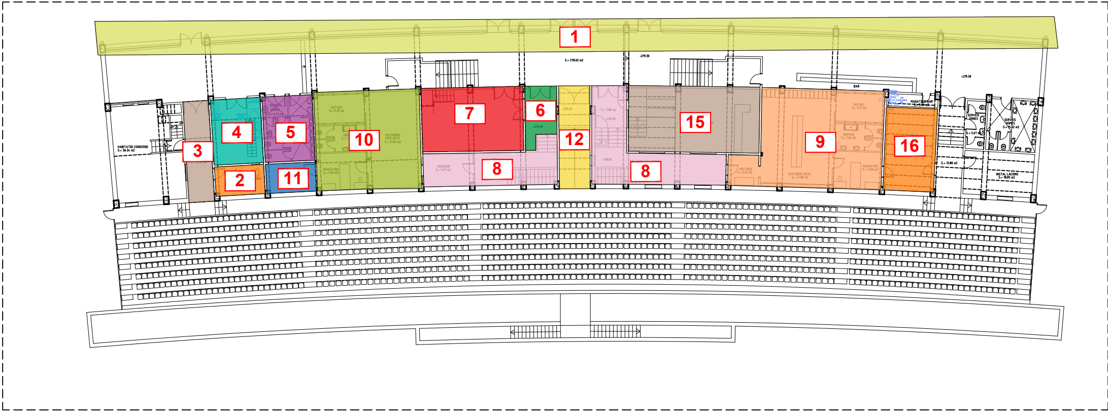
PLANTA BAIXA
