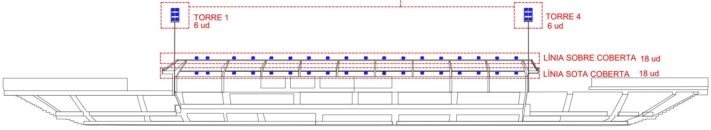
SECCIÓ A-A'
