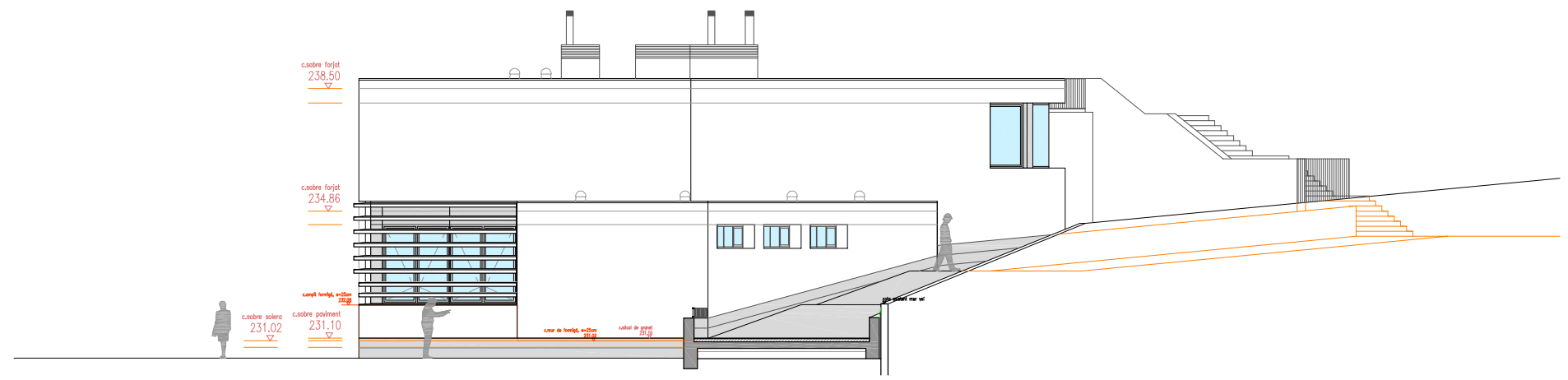
Alçat 1
