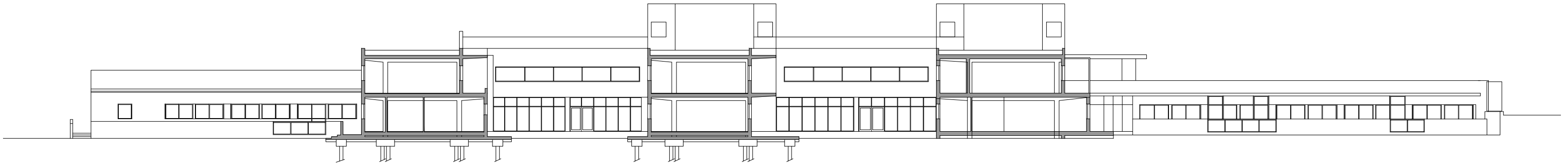
SECCIÓ LONGITUDINAL
