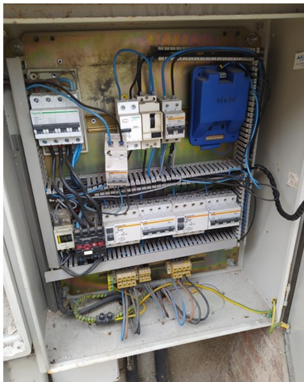
DETALL QUADRE ELÈCTRIC ENLLUMENAT PÚBLIC NÚM. 374
