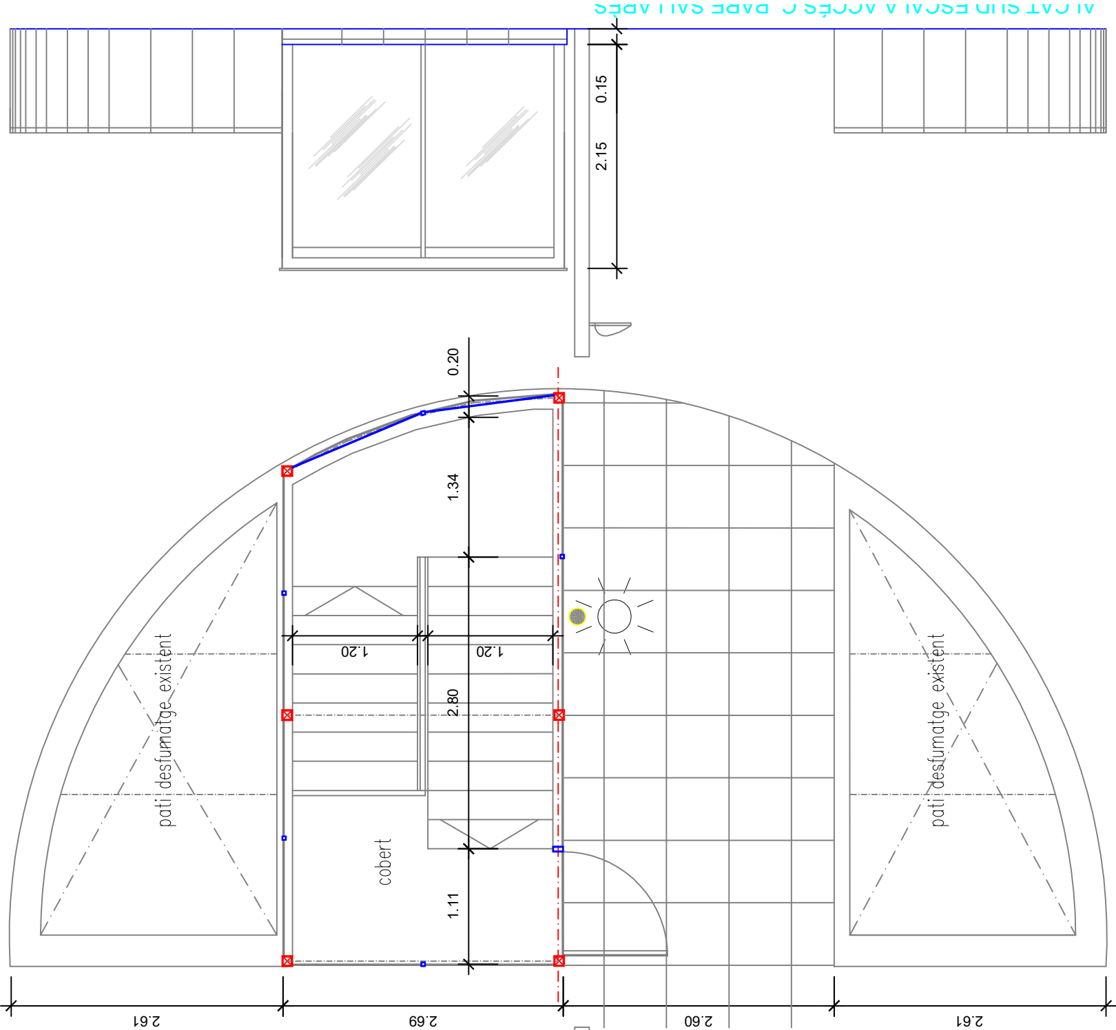
PLANTA ESCALA ACCÉS C. PARE SALLARÈS
