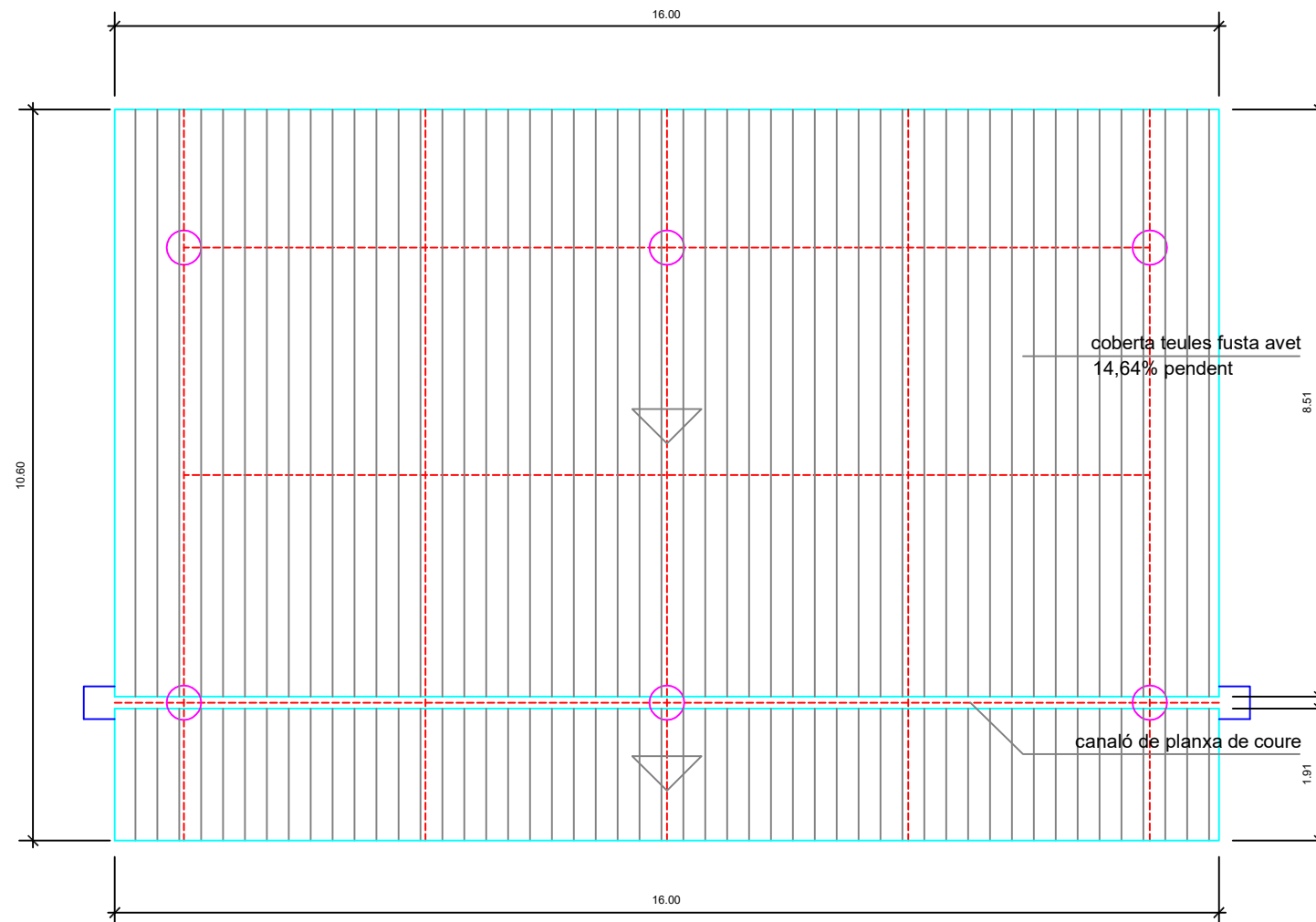
PLANTA COBERTA PORXADA Sup. coberta 169.60 m2
