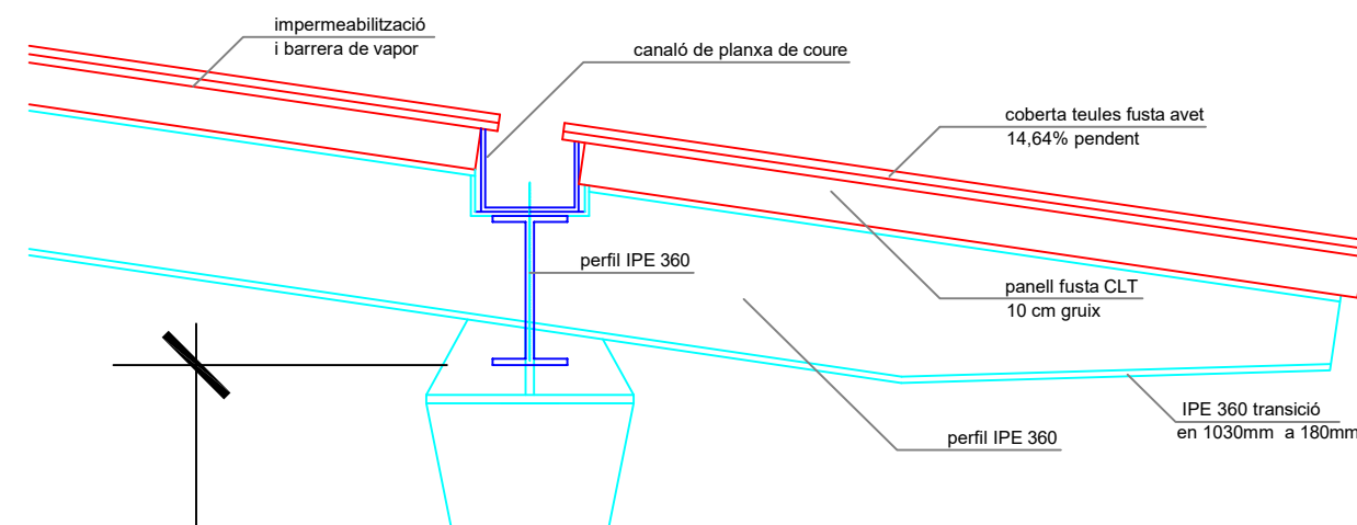
DETALL SECCIÓ COBERTA PORXADA E 1/20
