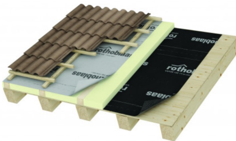
Sistema de coberta inclinada de fusta (en el nostre cas sense la capa d'aïllament tèrmic)
