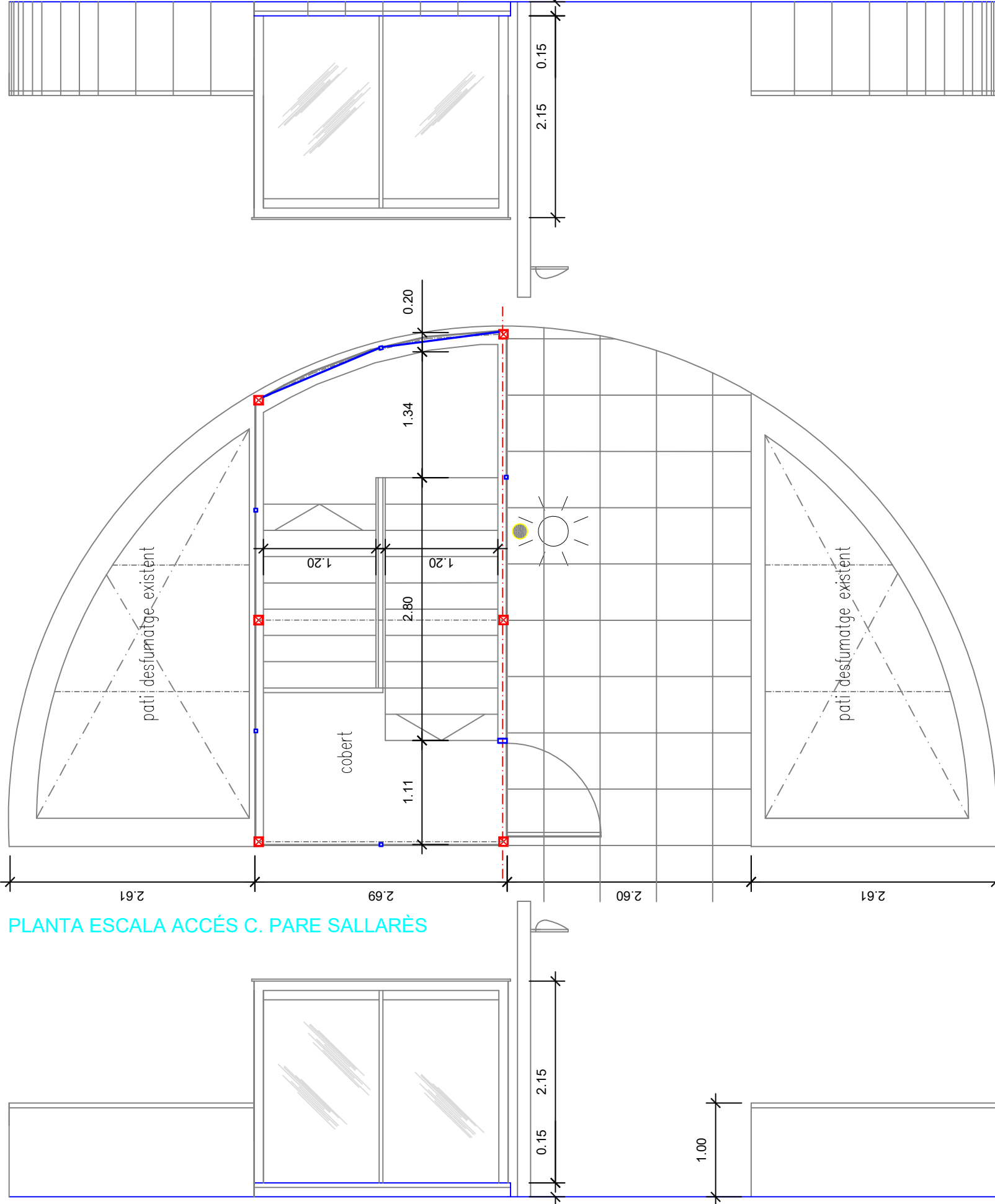
ALÇAT NORD ESCALA ACCÉS C. PARE SALLARÈS
