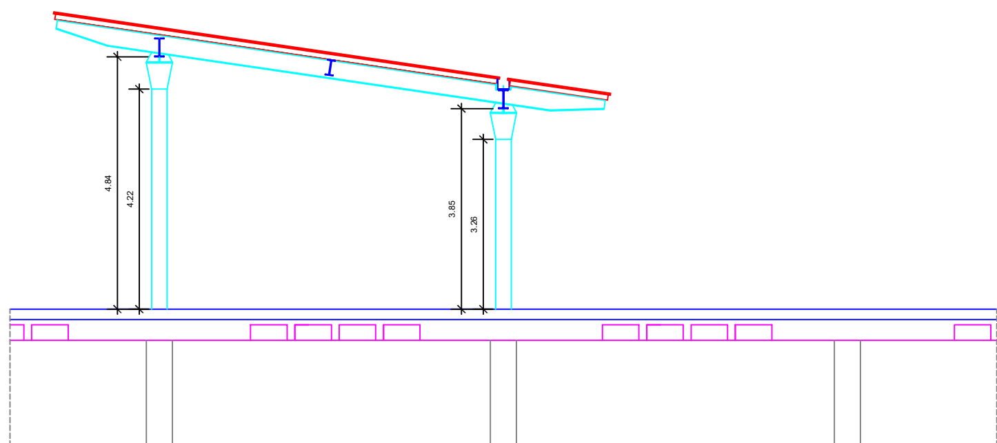
SECCIÓ PORXADA
