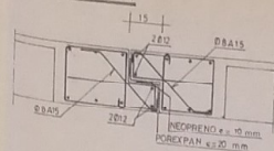
SECCION A-A
