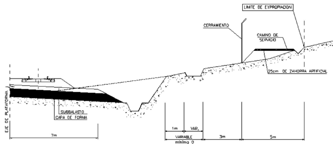
Figura 1. Esquema de disposición del camino de servicio y el cerramiento correspondiente
