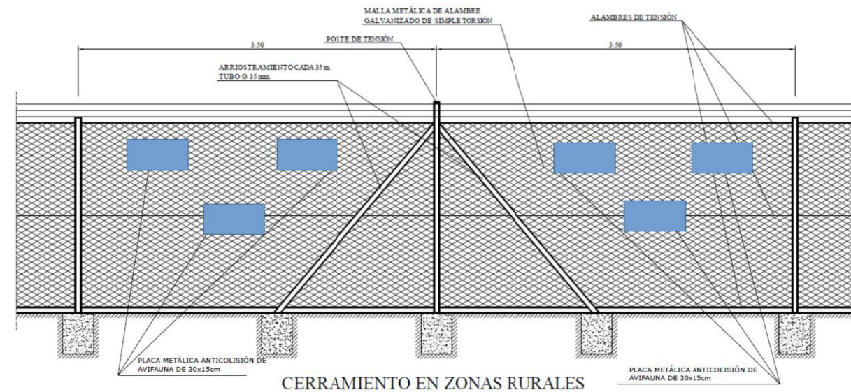
Figura 2. Esquema de cerramiento en zonas rurales.
