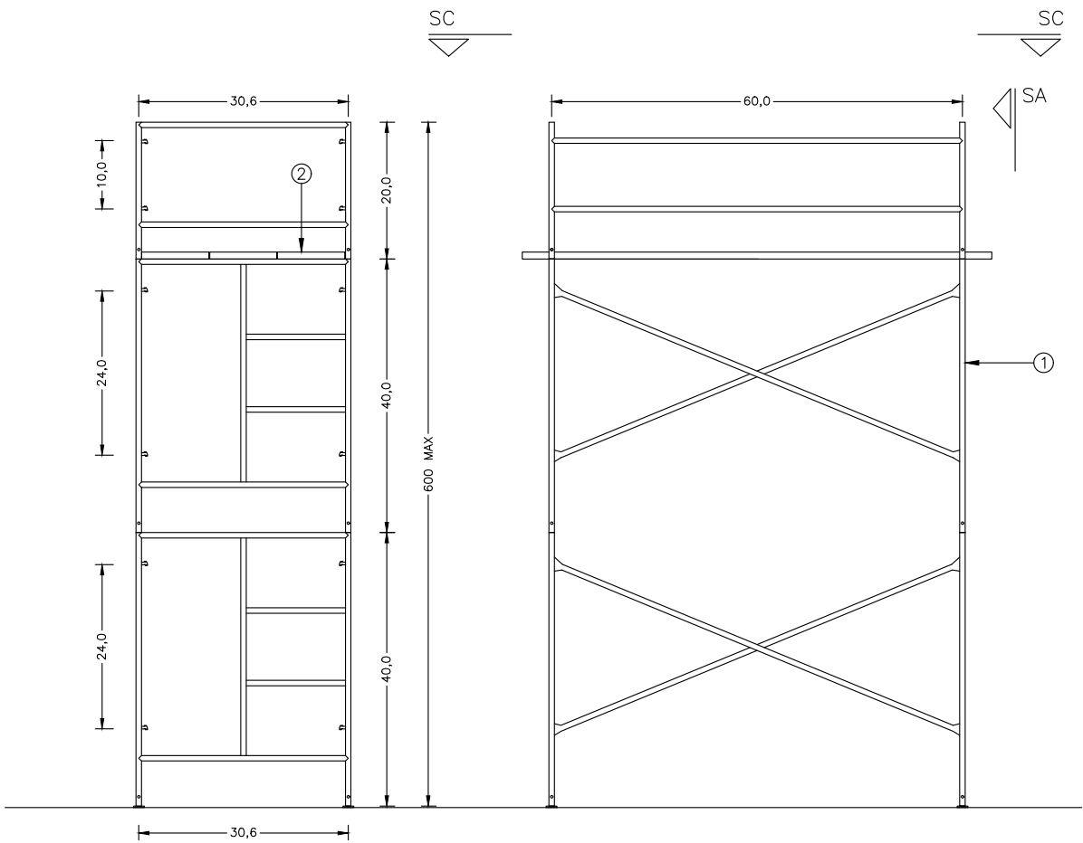
SECCIÓ A-A
