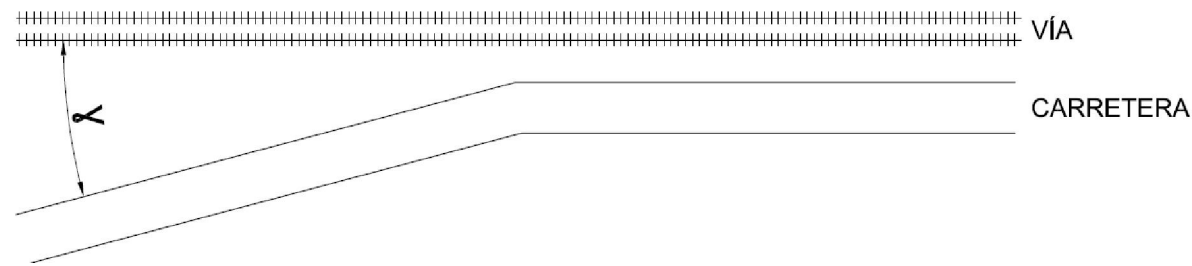
Figura 5. Ángulo de incidencia de los viales respecto a la traza ferroviaria.
