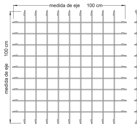
Fig: Ejemplo de enrejado monotec ®
