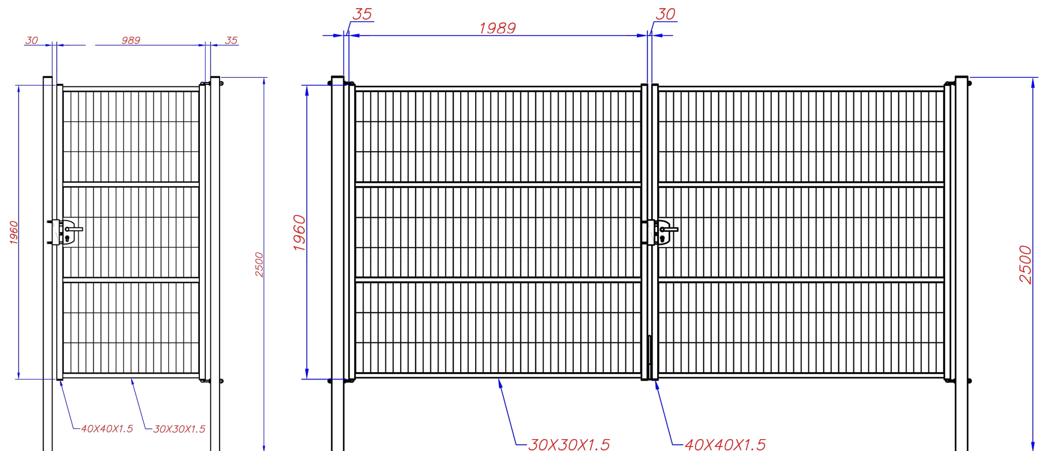
Suports, muntants, bastidor i malla electrosoldada d'acer galvanitzat en calente exterior i interior Z-275
