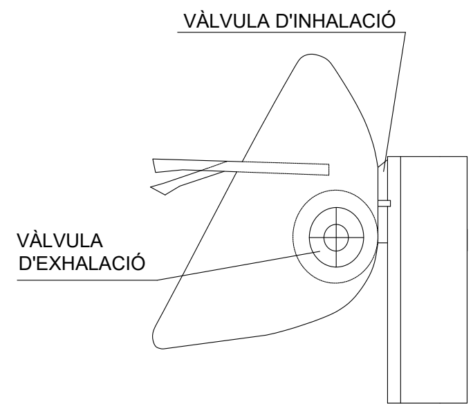
SECCIÓ A-A
