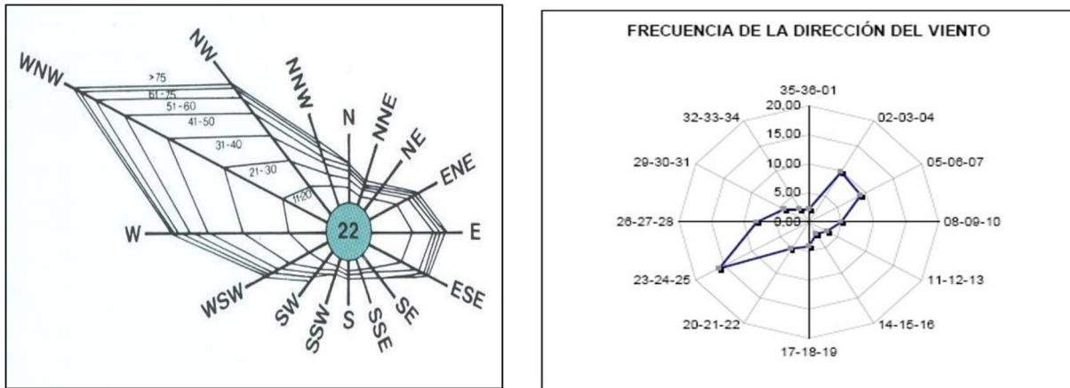
Figura 4. Ejemplo de rosas de los vientos.
