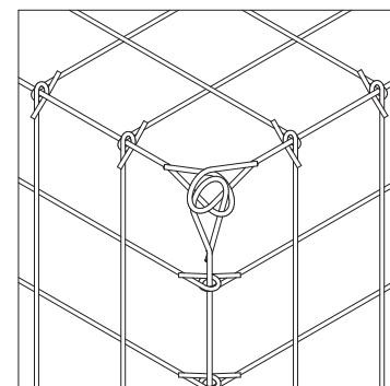
Fig: Cierres de empalme rápido correctamente unidos
