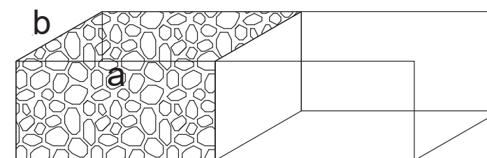
Fig: Primer gavión relleno
